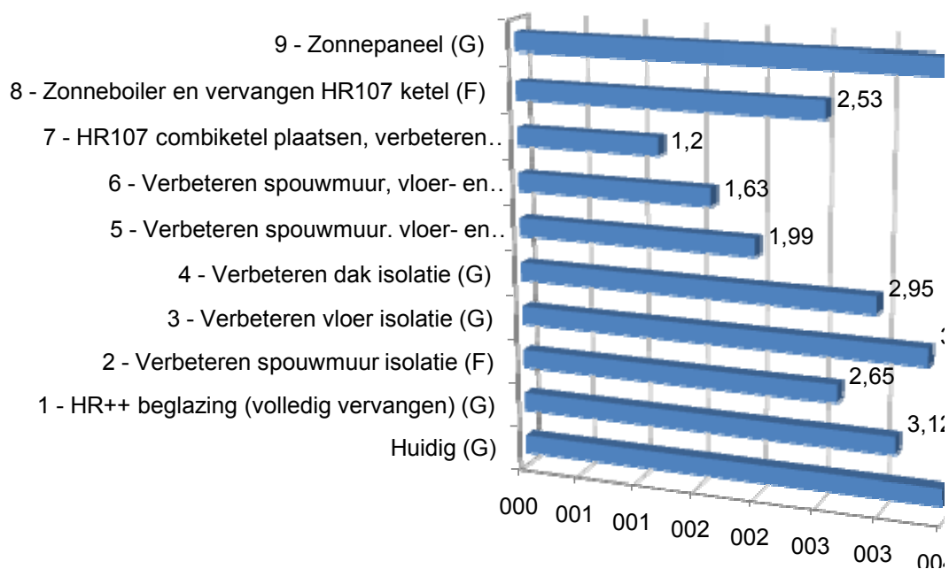
Energie-index per maatregelpakket
