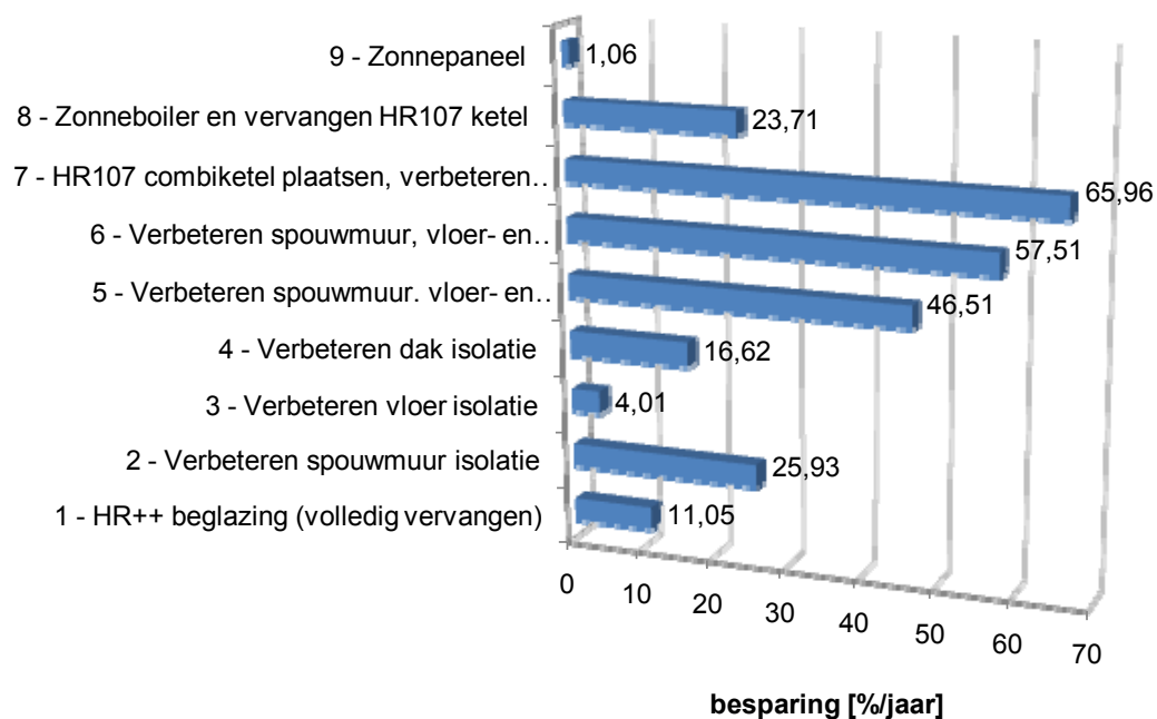
Energiebesparing per maatregelpakket
